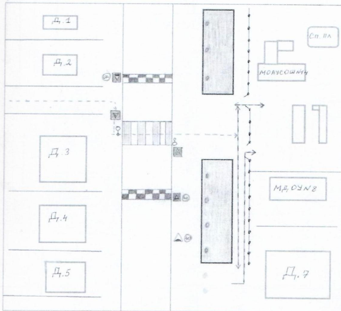
Схема организации дорожного движения в непосредственной близости от образовательного учреждения с размещением соответствующих технических средств, маршруты движения детей (учащихся) и расположение парковочных мест
